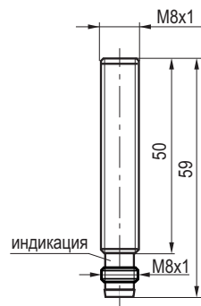
Габаритный чертёж
